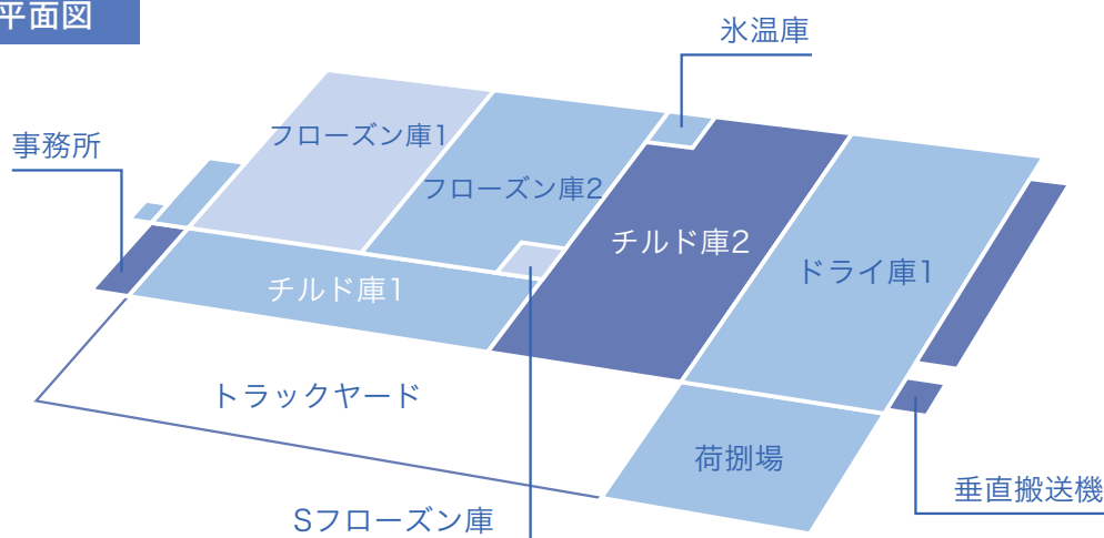
1階平面図
