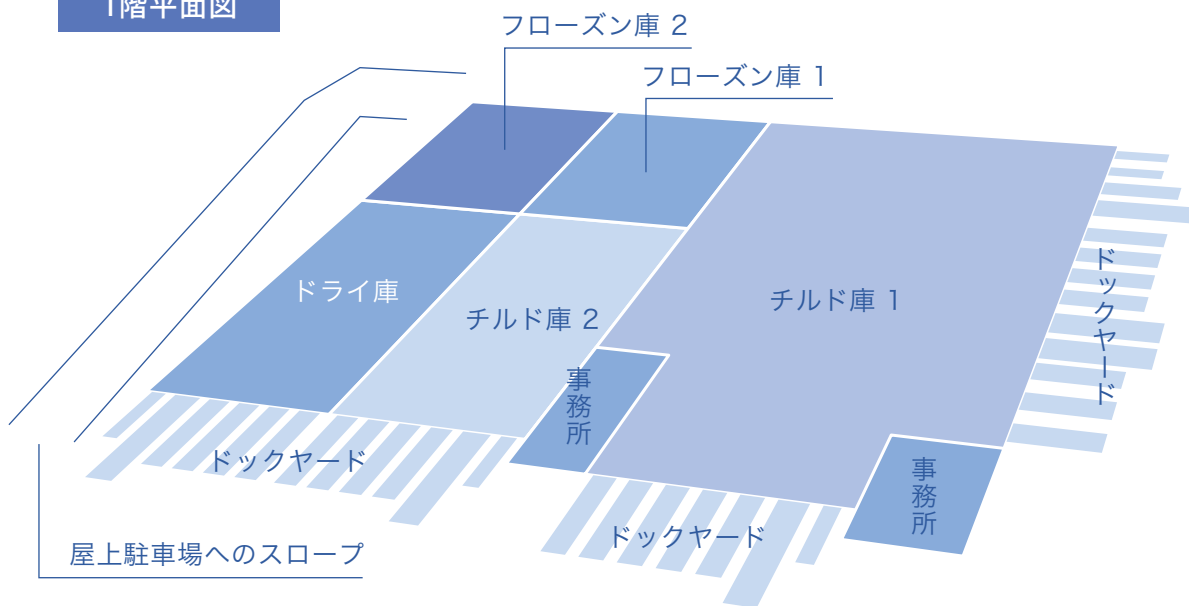
1階平面図
